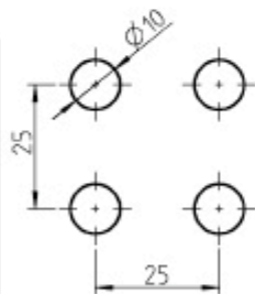
szablon otworu
