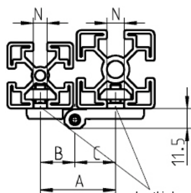
kostki do zamocowania w rowku
