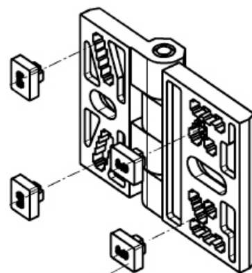
kostka do zamocowania w rowku
