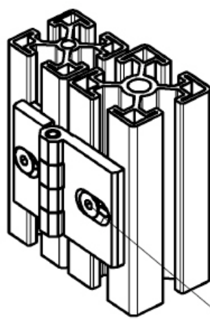
do śruby z łbem stożkowym M6 DIN 7991
