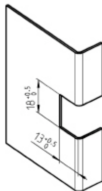
szablon otworu
