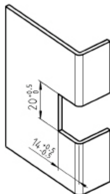
szablon otworu
